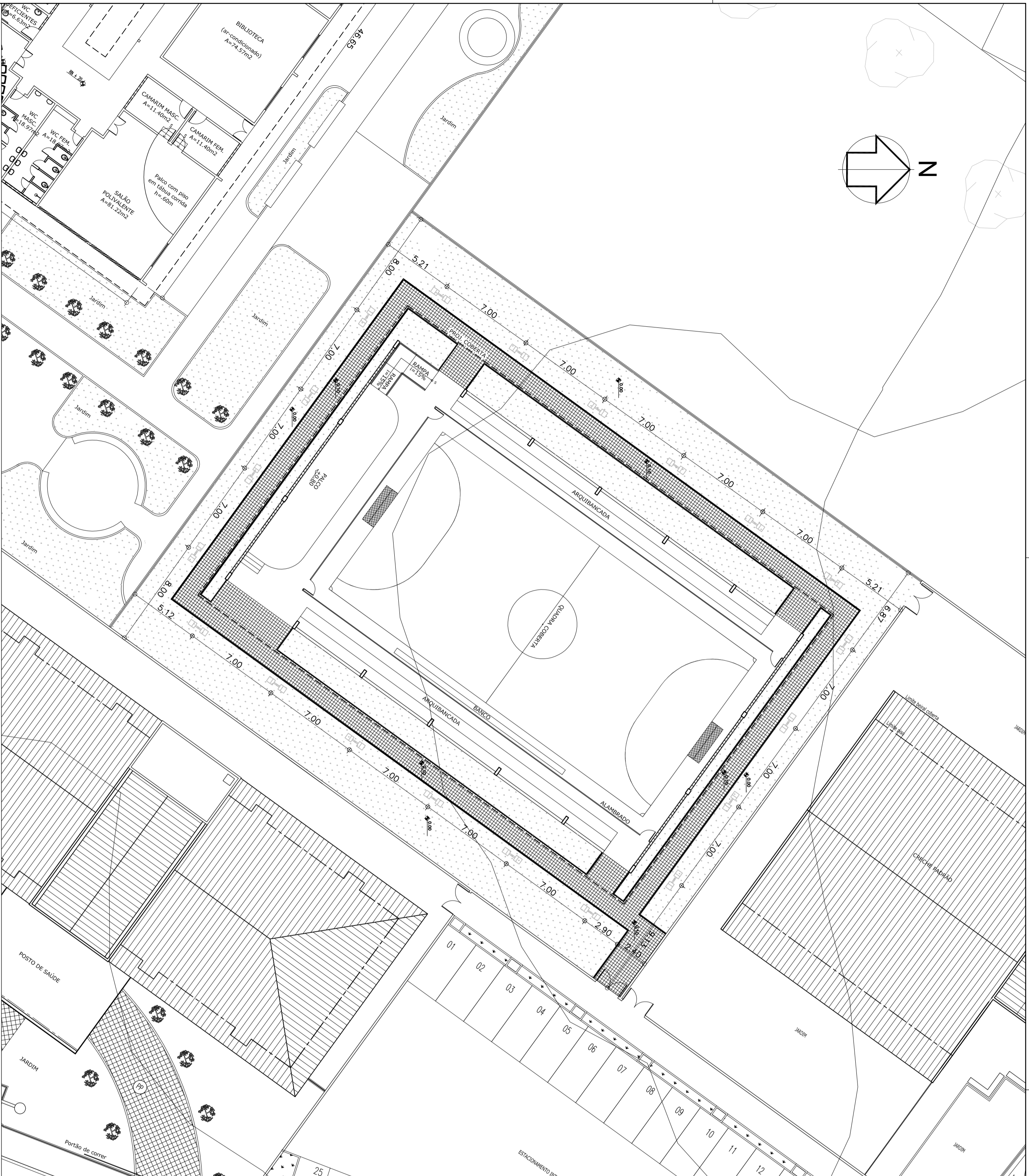
1 PLANTA DE ILUMINAÇÃO ESC.: 1:200
